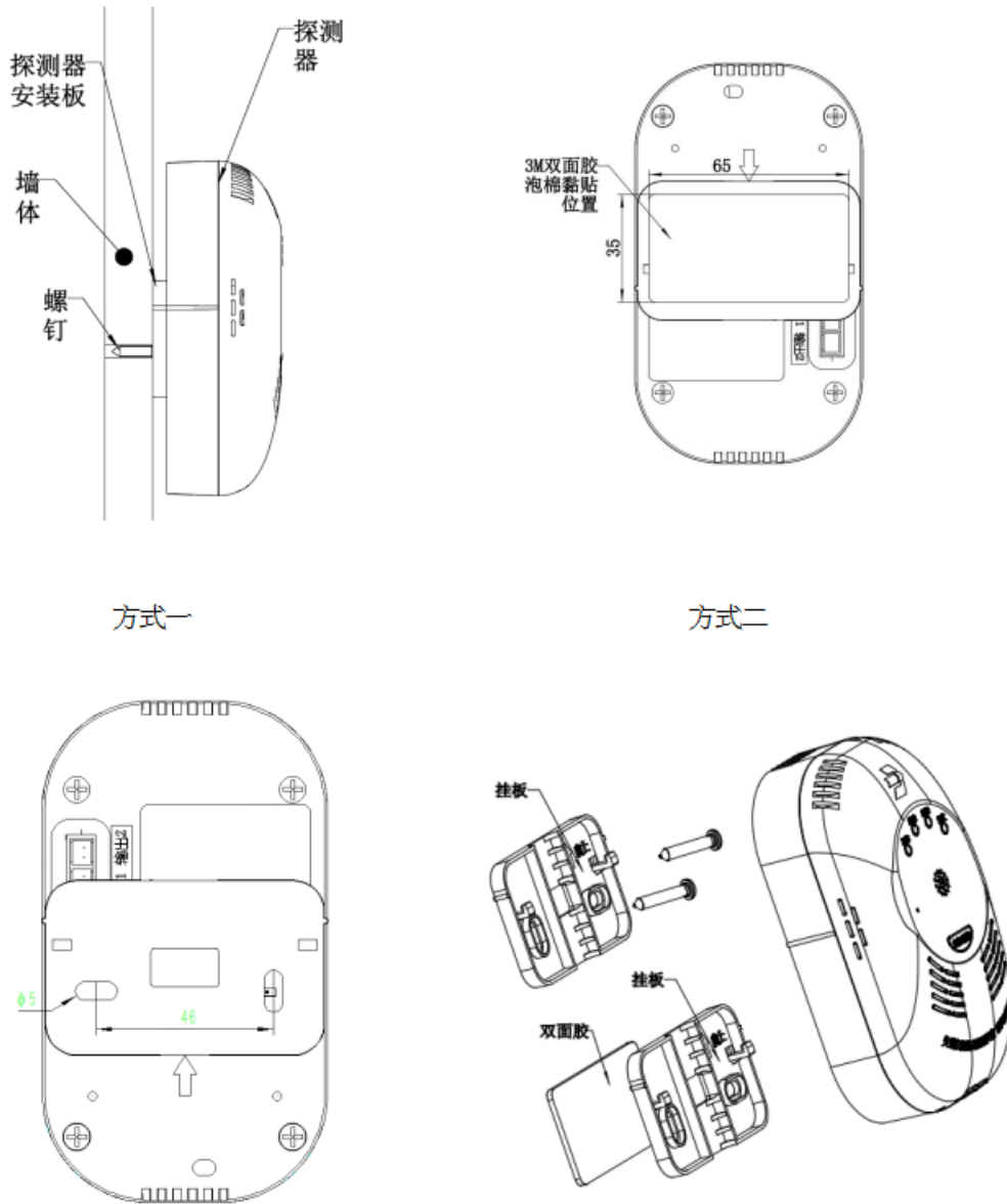
图 1 外形及安装尺寸图
