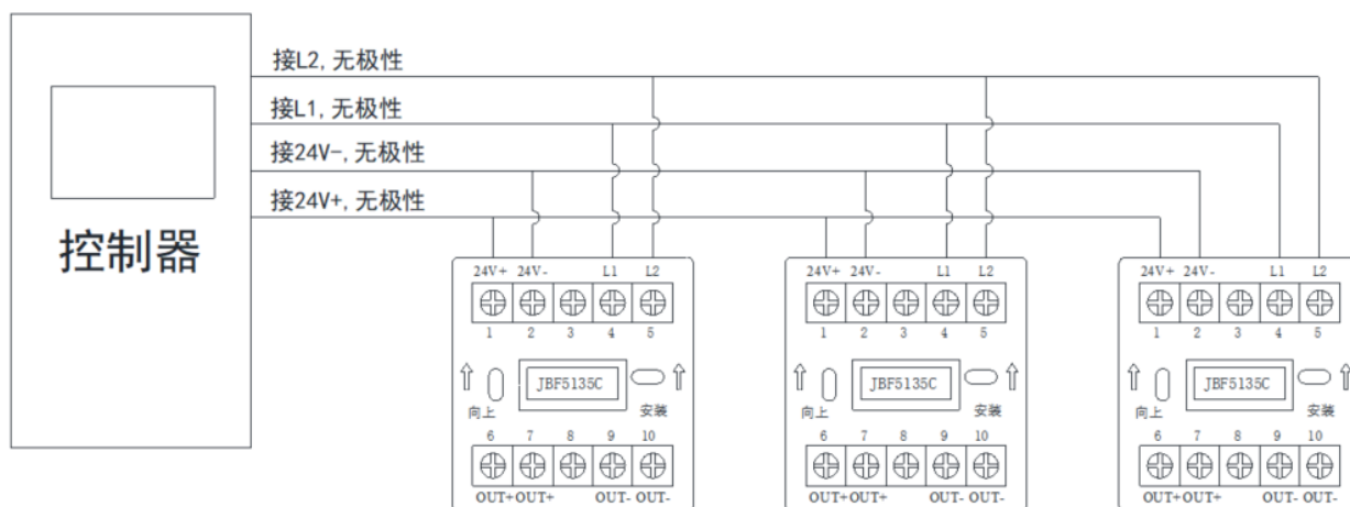
图 3 回路接线示意图
